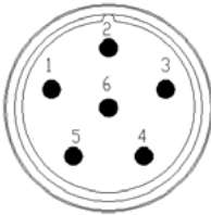
M23 电源插座 ( 额定电流 \leq 30\text{Arms} )
